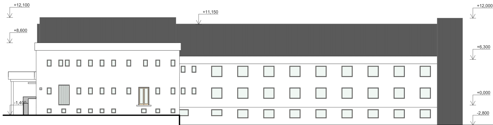
ZÁPADNÍ POHLED
